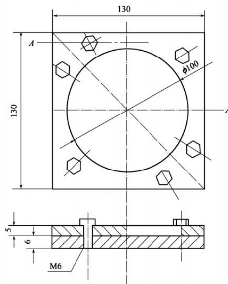
图 6 耐磨性制样器示意图
