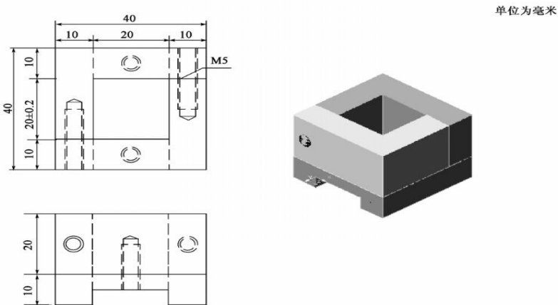
图 4 热熔型涂料密度制样器示意图
