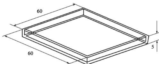
图 3 热熔型涂料色度性能制样器示意图
