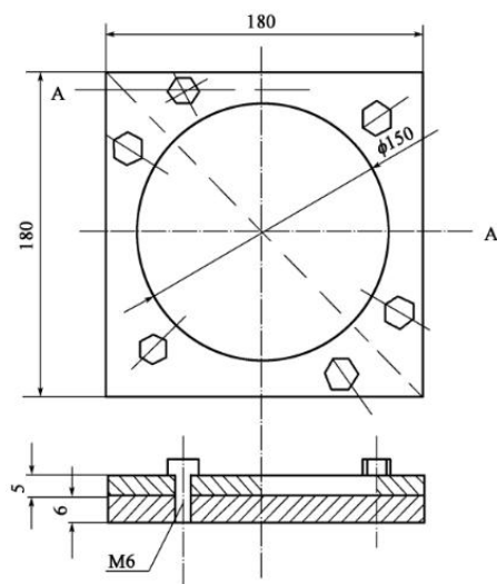
图 7 流动度制样器示意图
